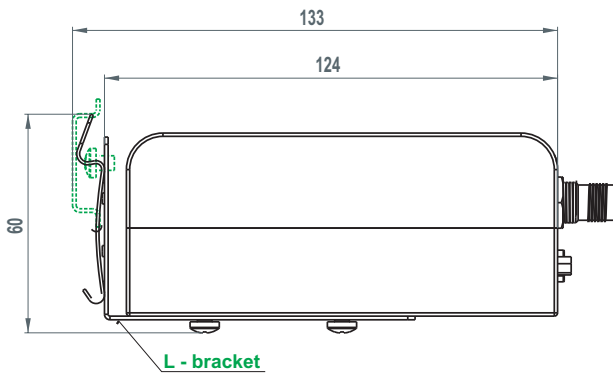
Fig. 5.19: RipEX.with L-bracket
