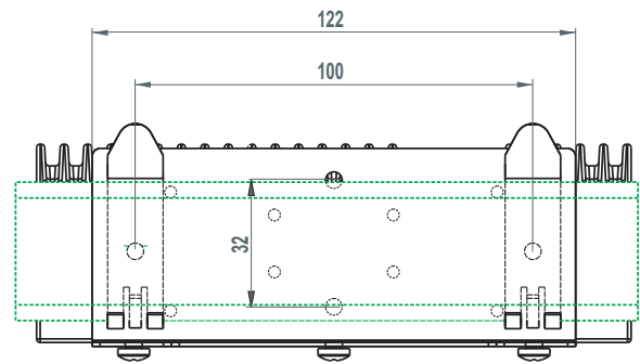
Fig. 5.18: L-bracket
