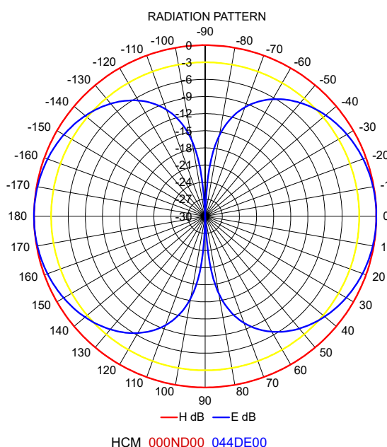
2300-5725 MHz
